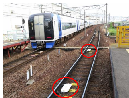
ATS地上装置
