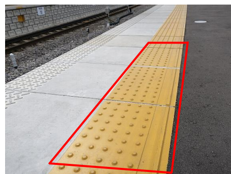
内方線付き点状ブロック
