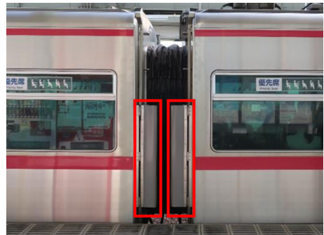
車両転落防止幌
