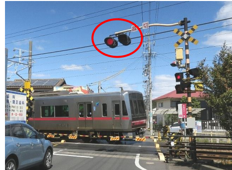
オーバーハングせん光灯
